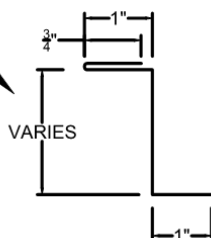
Z CLIP
